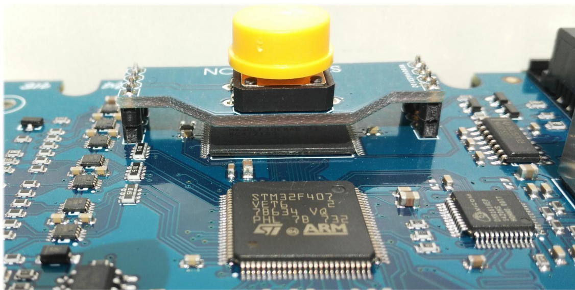
FLasher Pro V4 电路板 按键下的彩蛋
