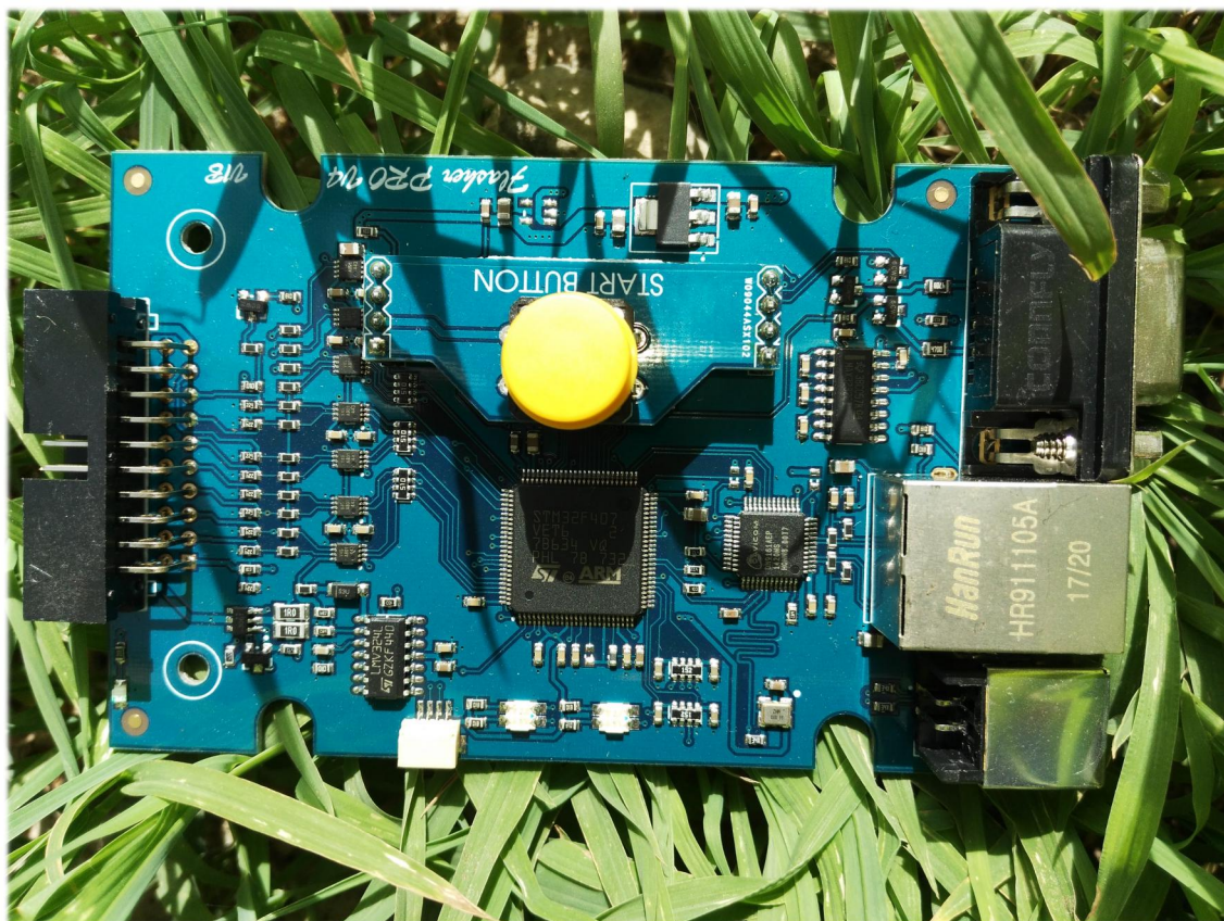
FLasher Pro V4 电路板 正面照
