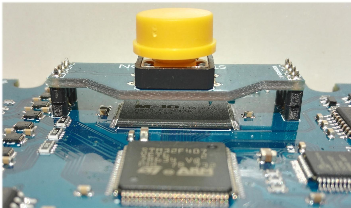
FLasher Pro V4 电路板 最大彩蛋
